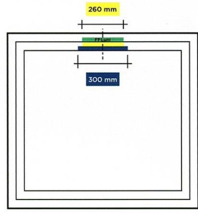
1 Stück Regel-air® FFLuni Variante für hohe Luftströme
