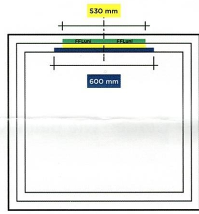
2 Stück Regel-air® FFLuni Variante für hohe Luftströme
